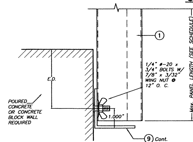
SECTION 1 STUD
